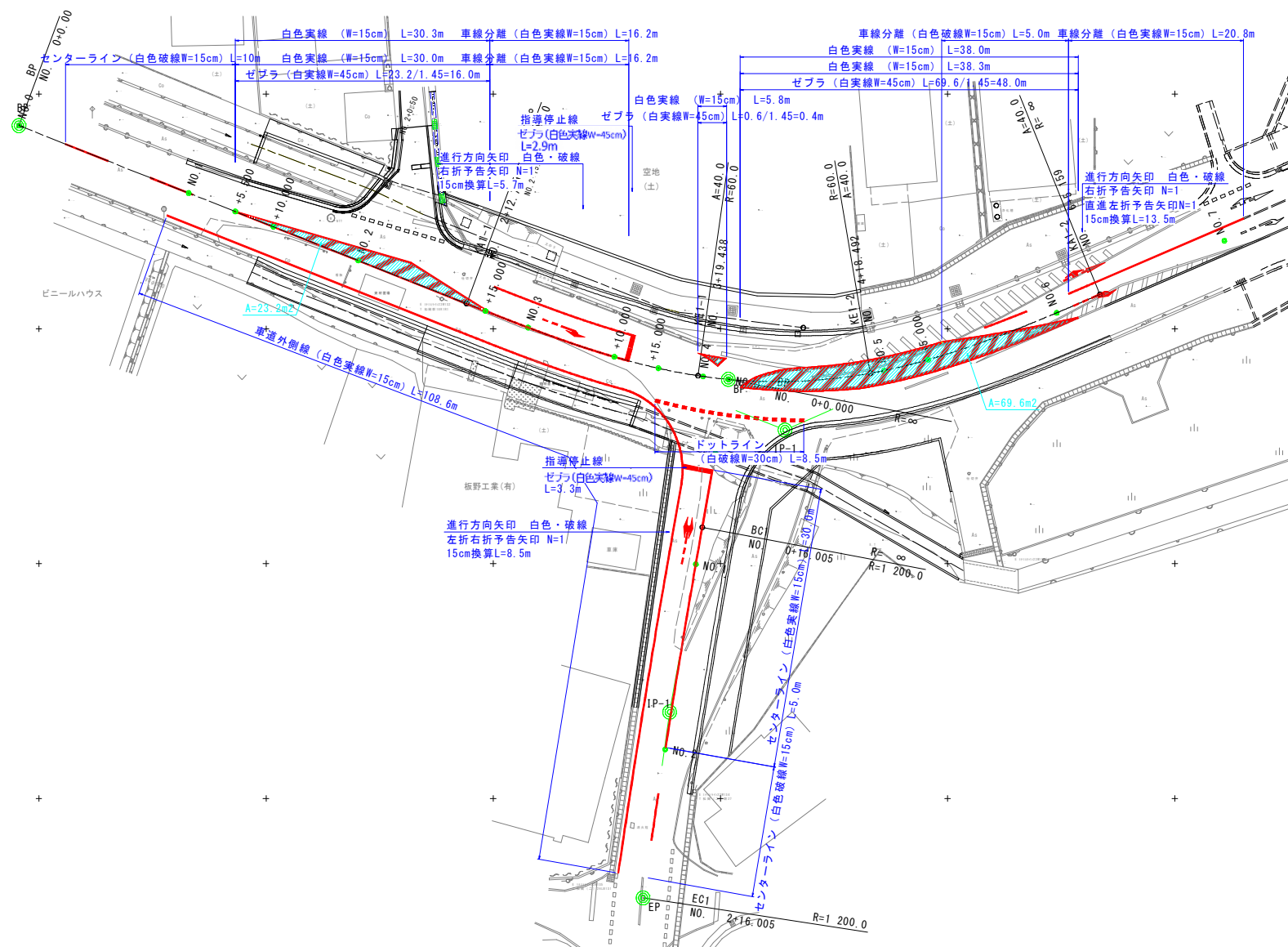
区画線数量算出根拠図
