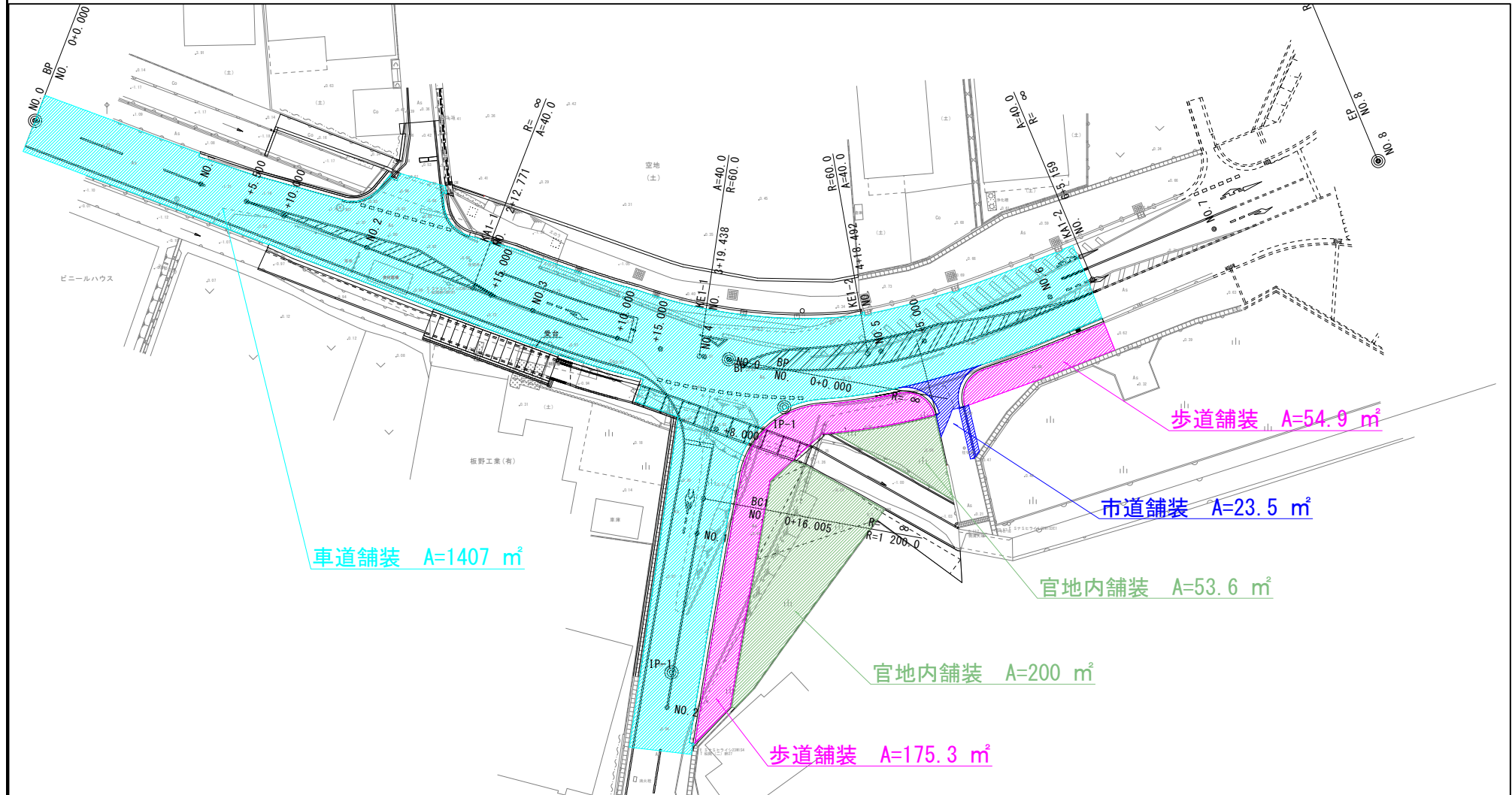
舗装面積算出根拠図
