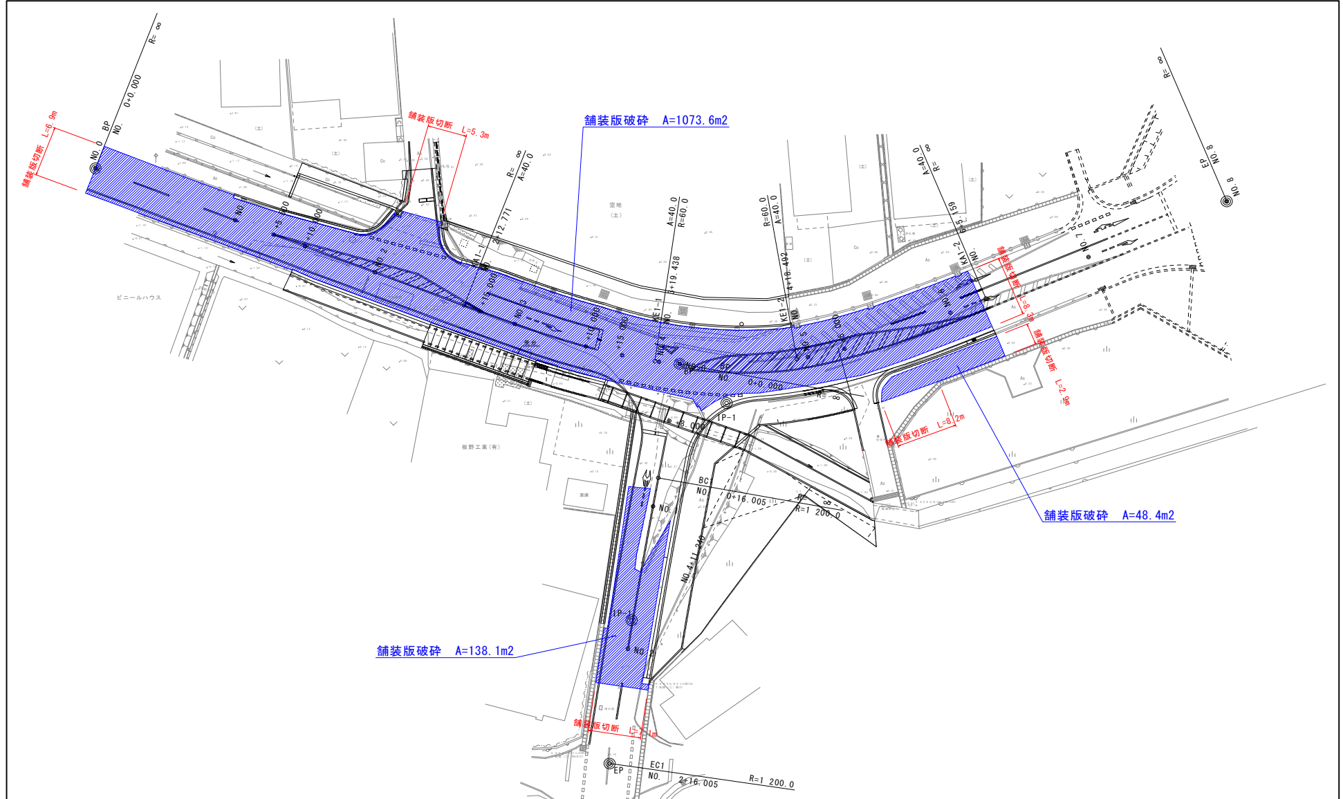
舗装取壊数量算出根拠図
